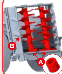
Streuwalzen Ø 820 oder 900 mm, je nach Modell, Windungen von 10 mm.
