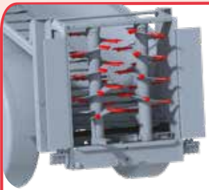
Austauschbare und wendbare Messerzinken aus HARDOX 450
